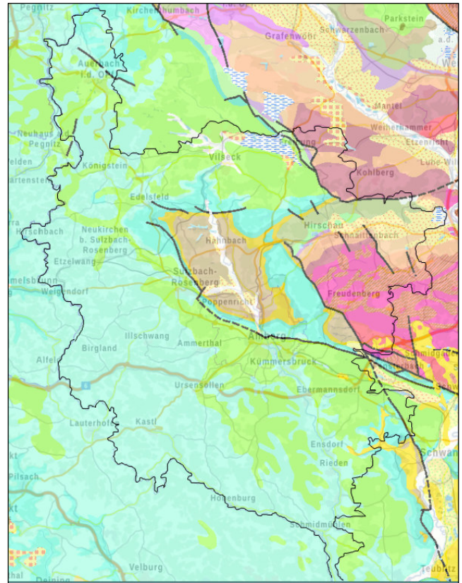
Abbildung 11: Geologische Karte für das LAG-Gebiet, Quelle: LfU
